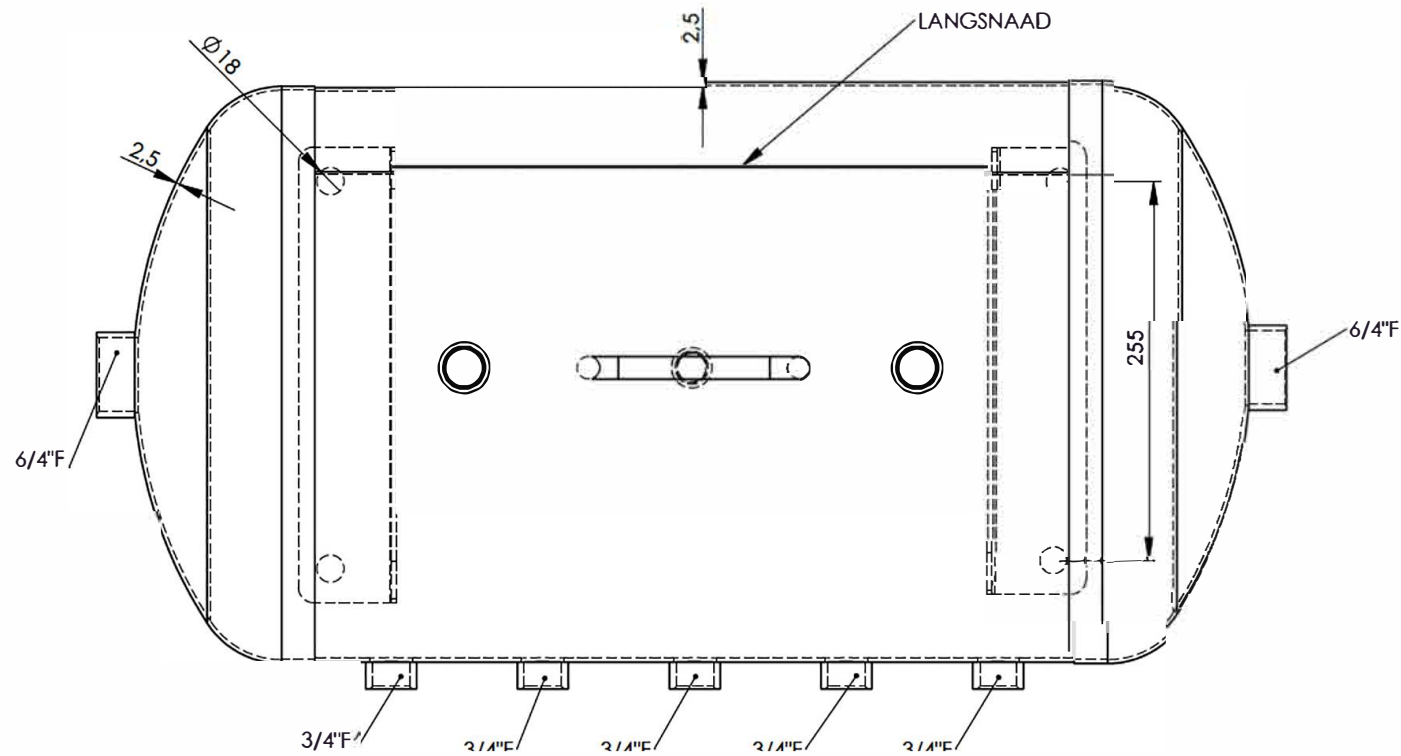
BOVENAANZICHT
